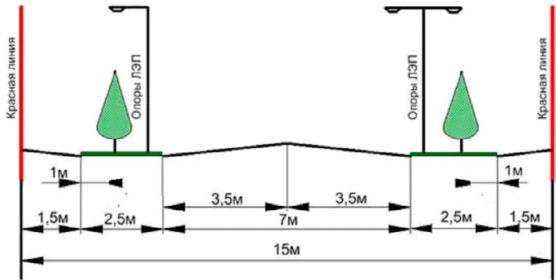
Поперечный профиль улицы
